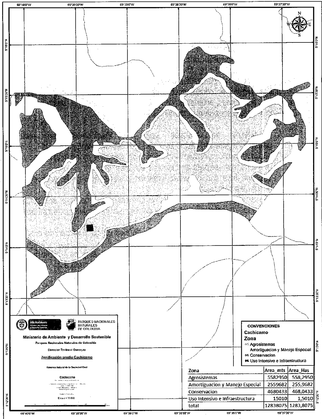
Mapa de Zonificación general del predio.
