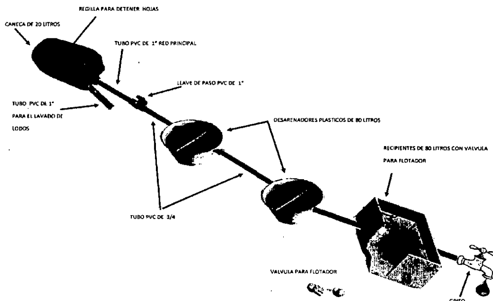
Figura 1. Sistema de captación propuesto
