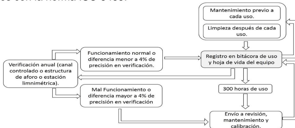
Figura 10. Diagrama de flujo del proceso de verificación y calibración de molinetes.
