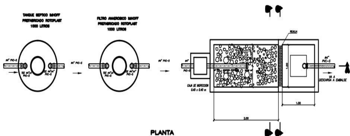
Figura 1. Diagrama del Sistema de Tratamiento. Fuente: Celsia Colombia S.A. E.S.P.-
