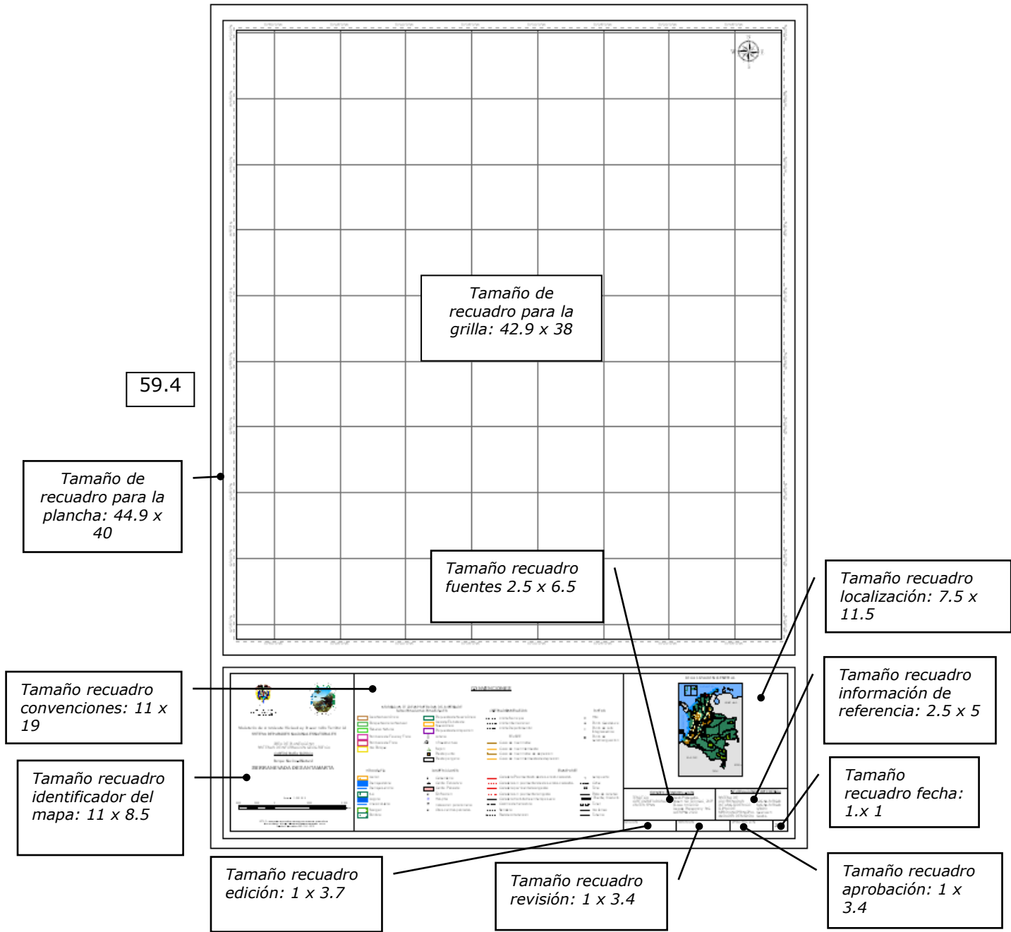
Figura 109: Tamaños de los apartes que componen el formato A2 vertical
