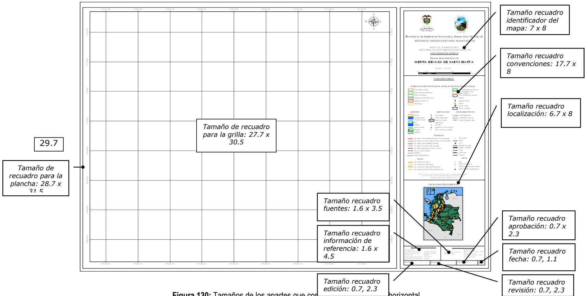
Figura 130: Tamaños de los apartes que componen el formato A0 horizontal
