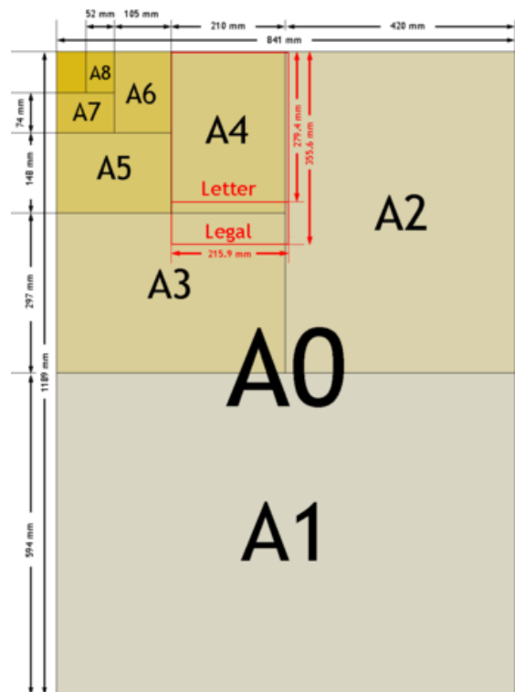
Figura 1: tamaños específicos para serie A de norma ISO216
