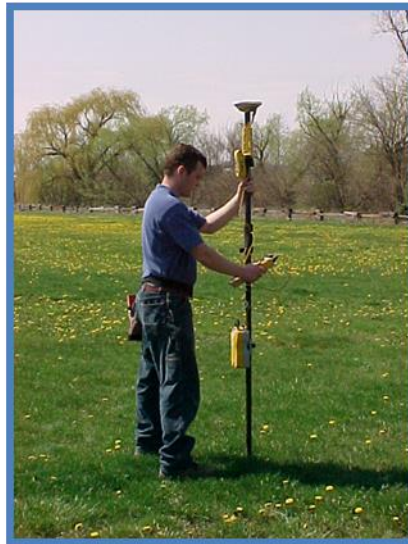
Ilustración 15 Equipo móvil "rover"
