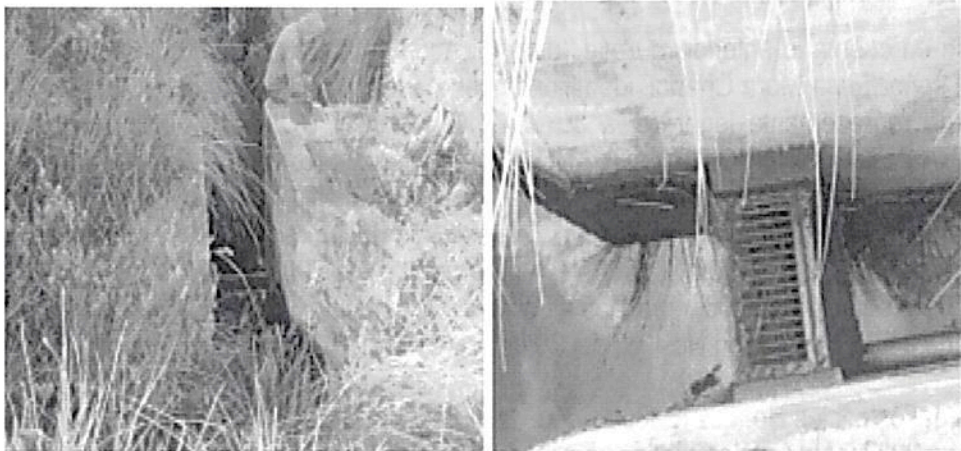
Imagen 1: Bocatoma Acueducto La Pradera. Fuente. Informe de seguimiento 13 de octubre de 2022
