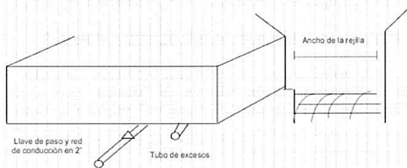
Imagen 2: Sistema de captación. Fuente. Informe de seguimiento 13 de octubre de 2022
